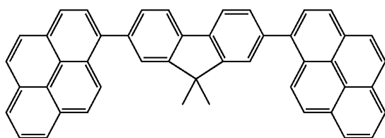
DFDP
