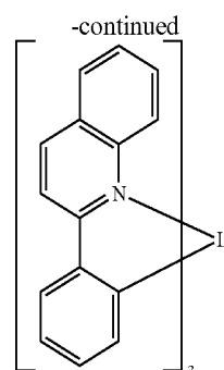
Ir(2-phq) 3
